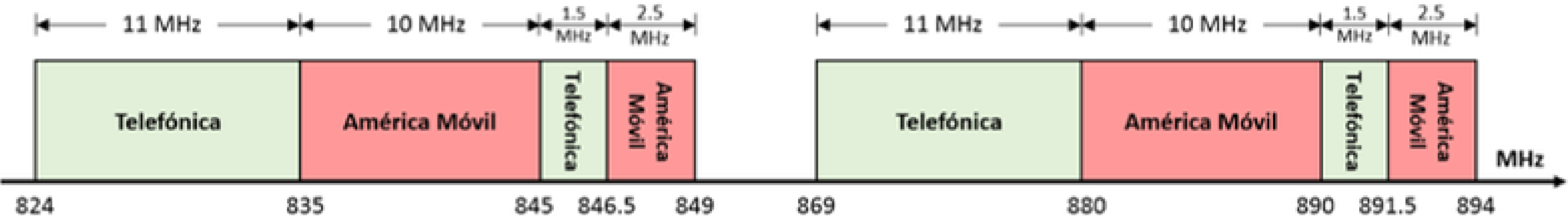
Figura N° 64.- Banda de 850 MHz
