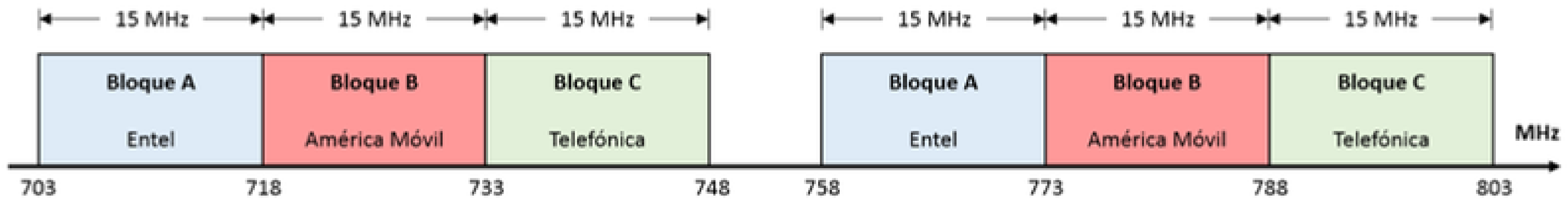
Figura N° 62.- Banda de 700 MHz
